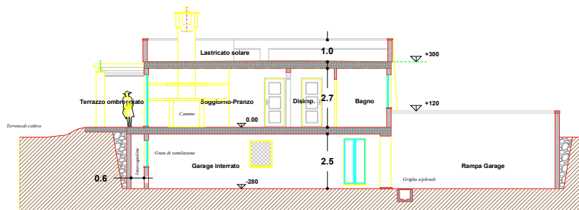
Sezione A-A'
