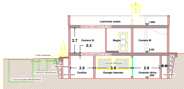
Sezione B-B'
